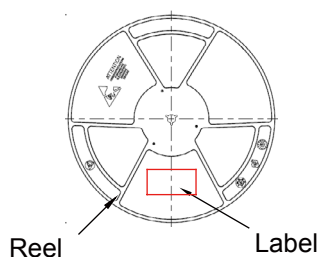
Taping reel dimensions
